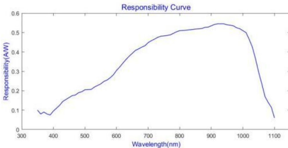
探测器响应度曲线
