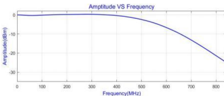
探测器频率响应曲线
