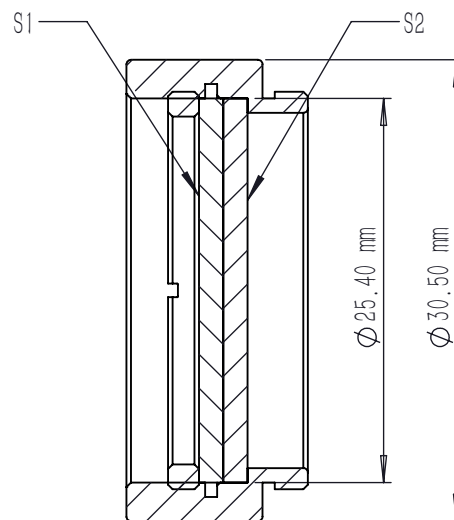
剖面 A-A
