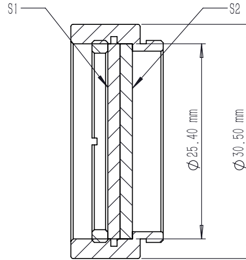
剖面 A-A
