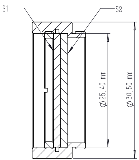
剖面 A-A
