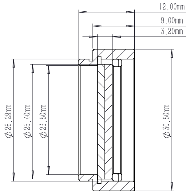
剖面 A-A
