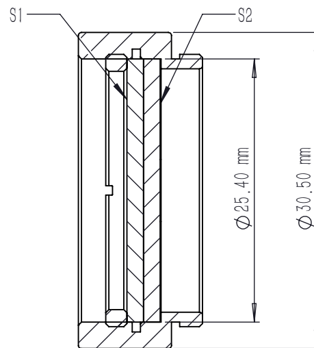
剖面 A-A
