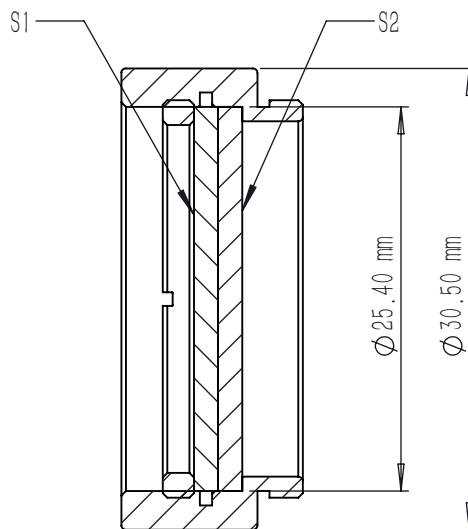
剖面 A-A
