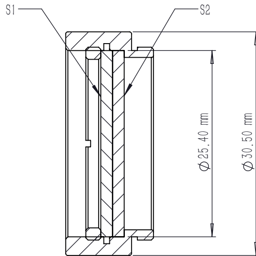
剖面 A-A
