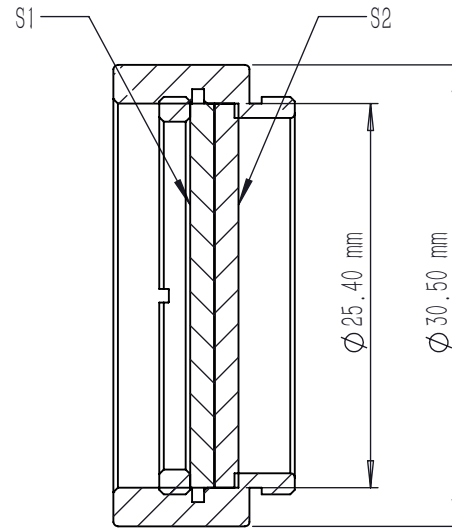
剖面 A-A
