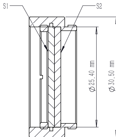
剖面 A-A
