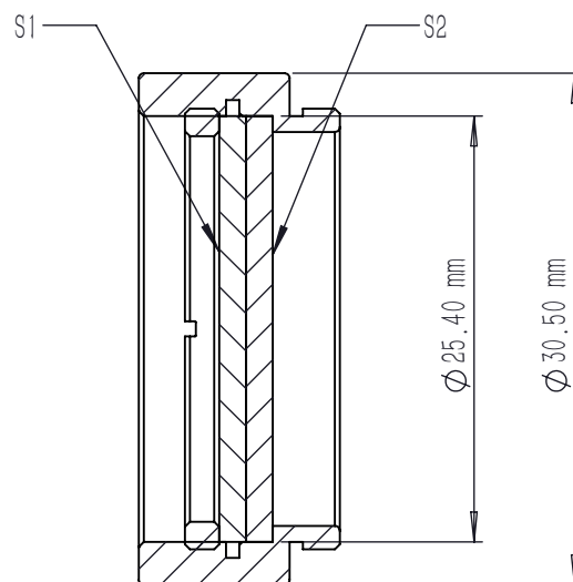
剖面 A-A
