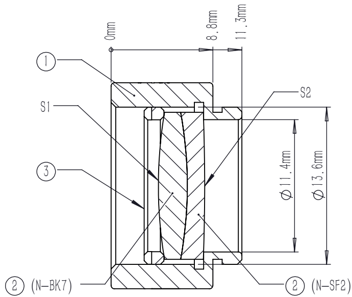
剖面 A-A
