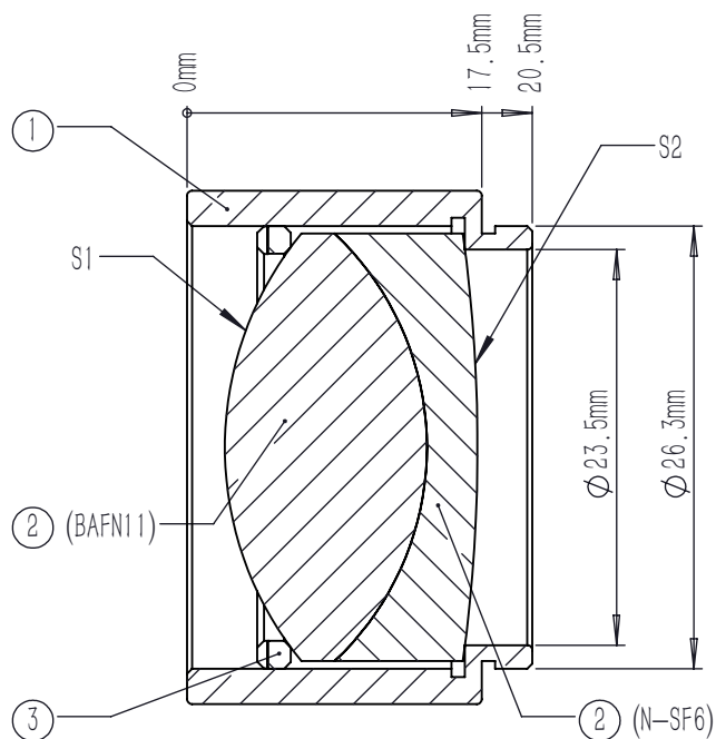
剖面 A-A
