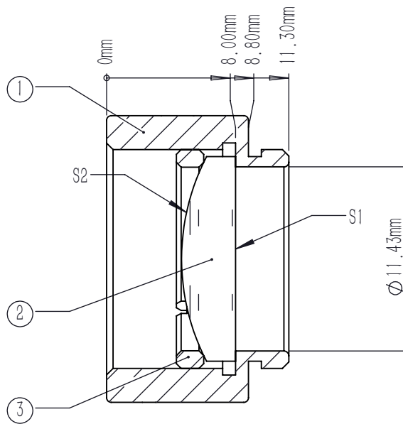
剖面 A-A
