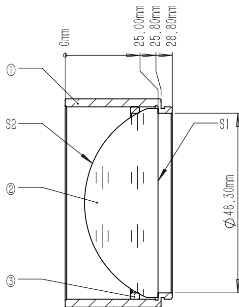
剖面 A-A
