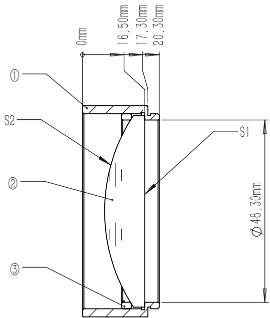
剖面 A-A
