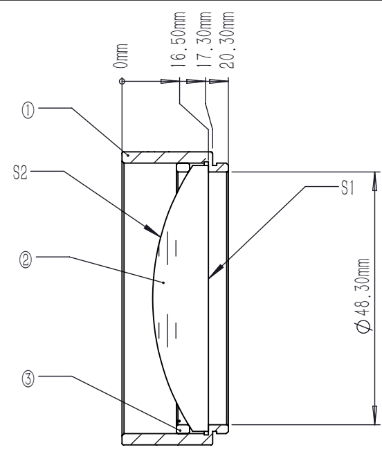
剖面 A-A
