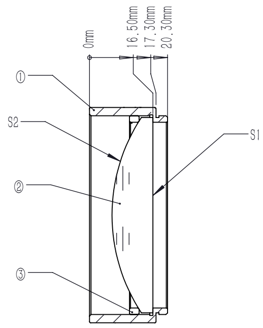
剖面 A-A
