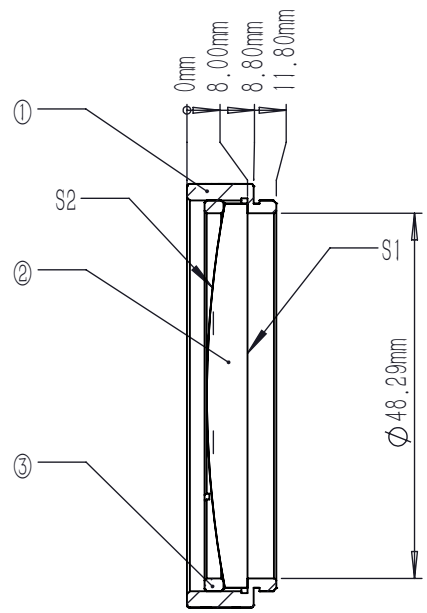
剖面 A-A
