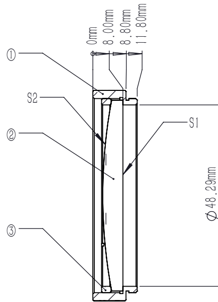
剖面 A-A
