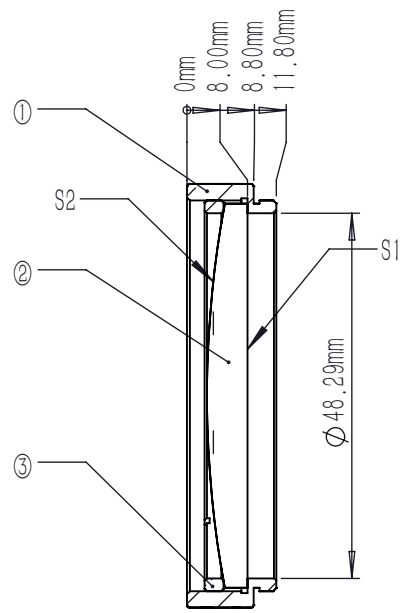
剖面 A-A
