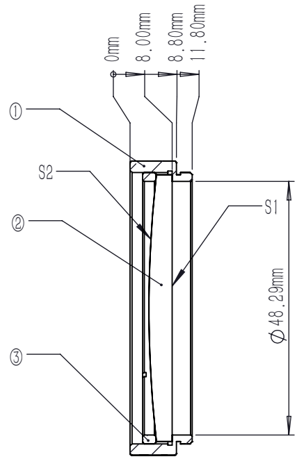
剖面 A-A
