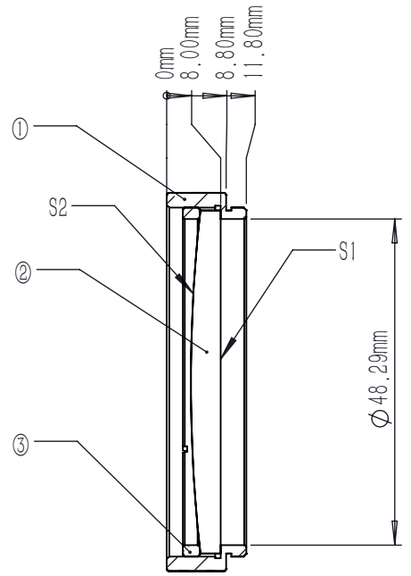
剖面 A-A
