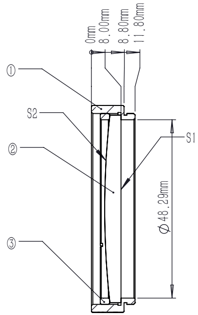
剖面 A-A
