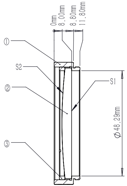
剖面 A-A
