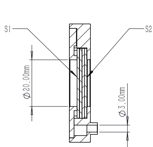
剖面 A-A
