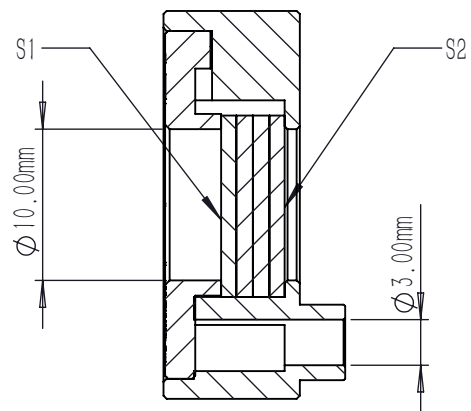
剖面 A-A
