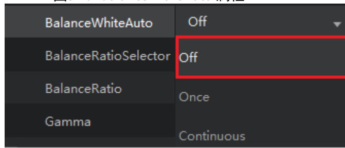
图3-29 BalanceWithAuto 属性
