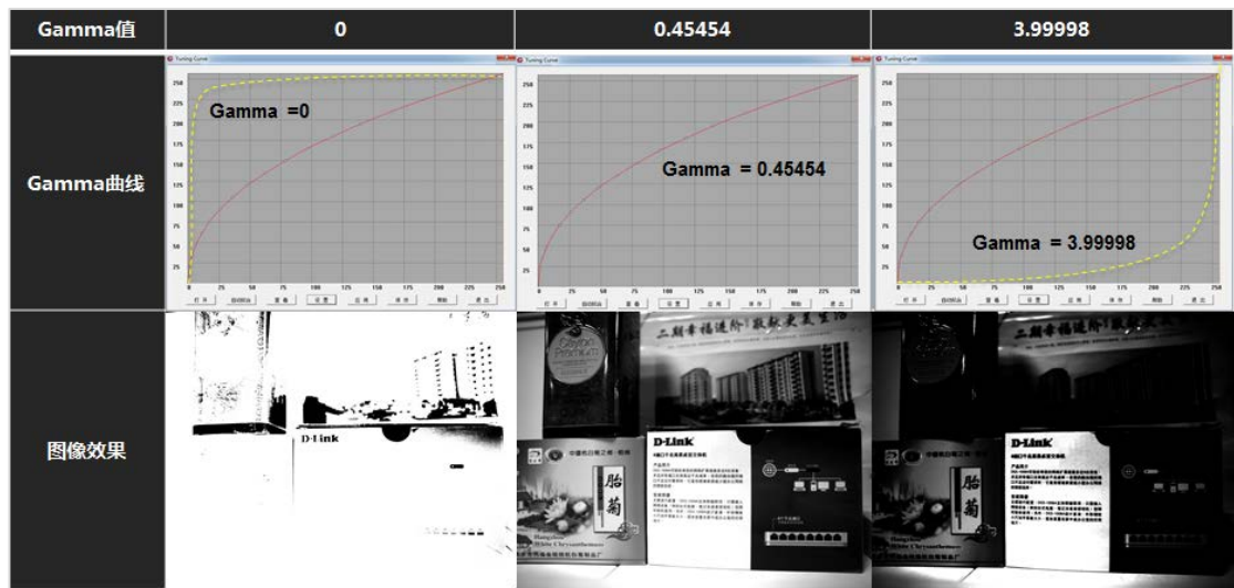
图3-32 Gamma 值
