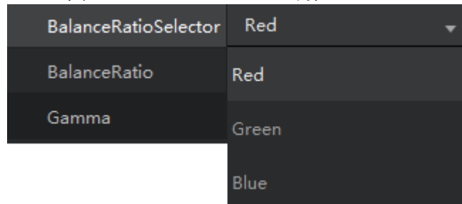
图3-30 BlackRatioSelector 属性
