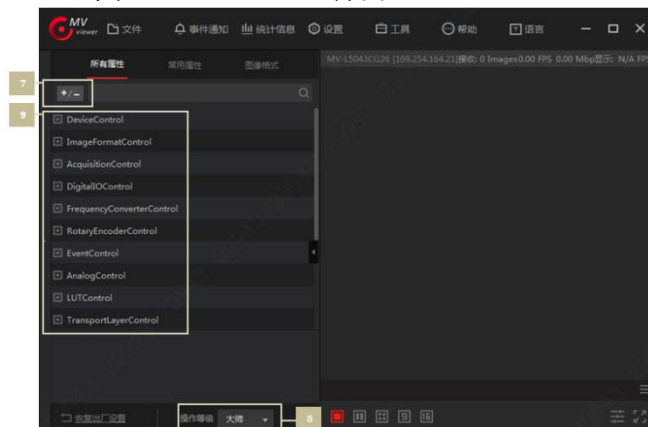
图2-2 MVViewer 主界面（2）
